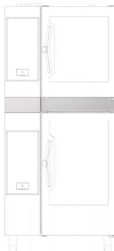
Sada pro instalaci konvektomatu 6 GN 1/1 na 6&10 GN 1/1 el., V = 120 mm
